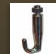
Крючок «Captain hook» На леску - до 10 кг На трос - до 15 кг CH-425
