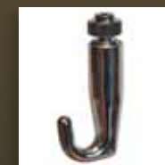
Крючок «Captain hook» На леску - до 10 кг На трос - до 15 кг CH-425
